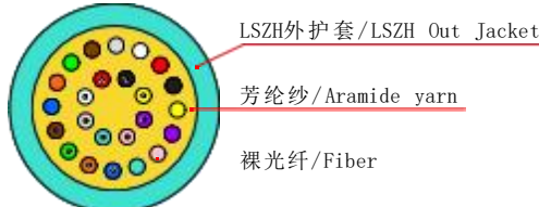
光缆示意图 Optical cable Diagram
