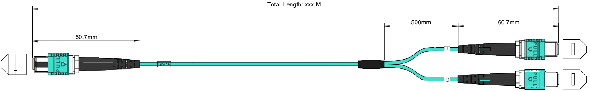
光缆示意图 Optical cable Diagram
