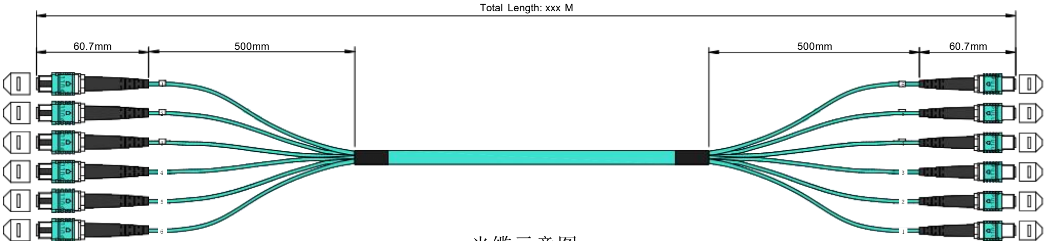
光缆示意图 Optical cable Diagram
