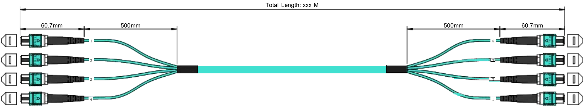
光缆示意图
