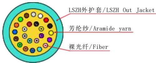
光缆示意图 Optical cable Diagram
